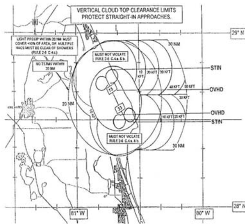
Fig. 12 Final Thunderstorm Overlay (NASA, 1996).
