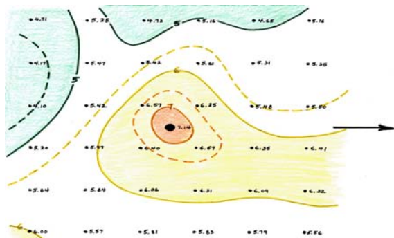
c. 850-500 mb
